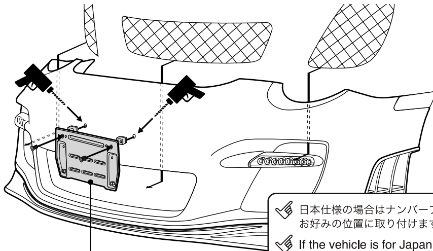
ナンバープレート・ステー (日本のみ) / License plate stay (Only in Japan)
