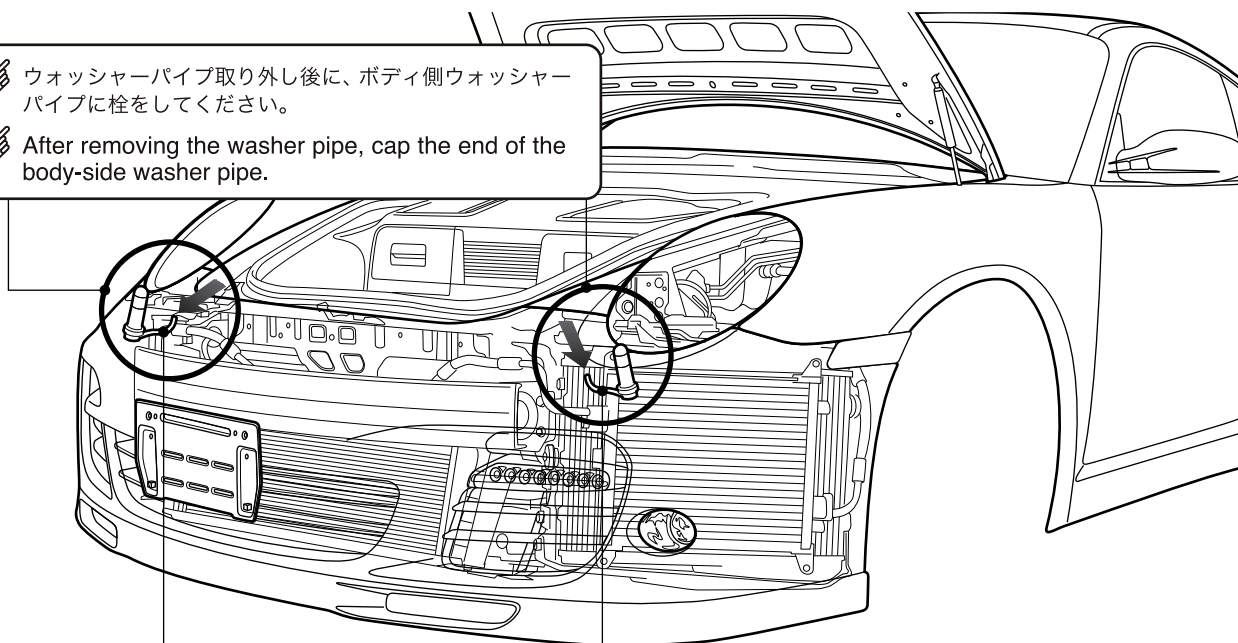
ウォッシャーパイプ / Washer Pipes
