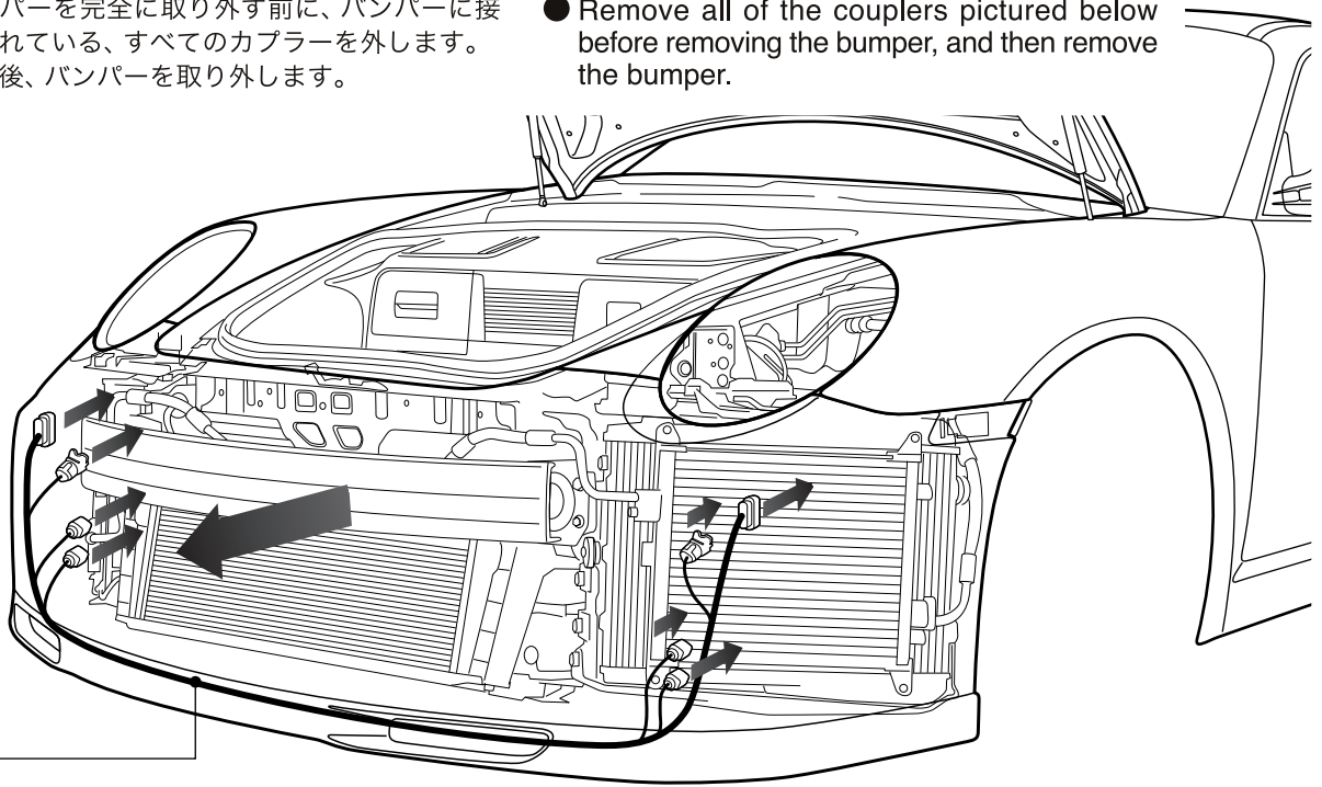
ハーネス / Harness
